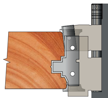
Single Door Edge
