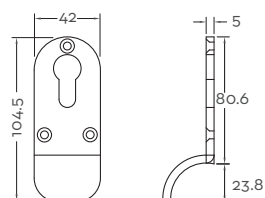
Internal Cylinder Pull (used in SE40A & SE40D)
